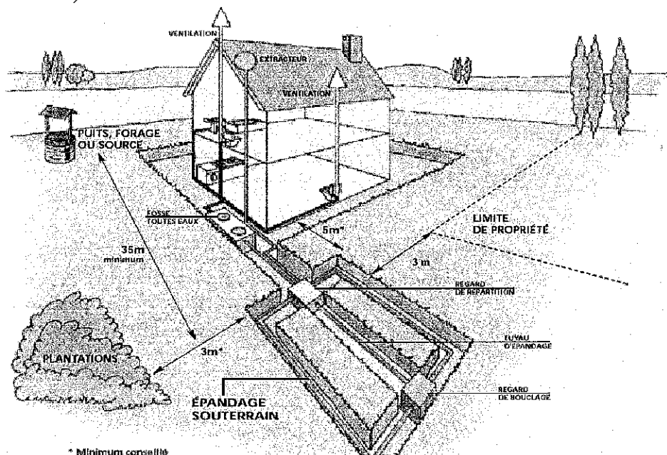
* Minimum conseillé Schéma général d'un dispositif d'assainissement non collectif
