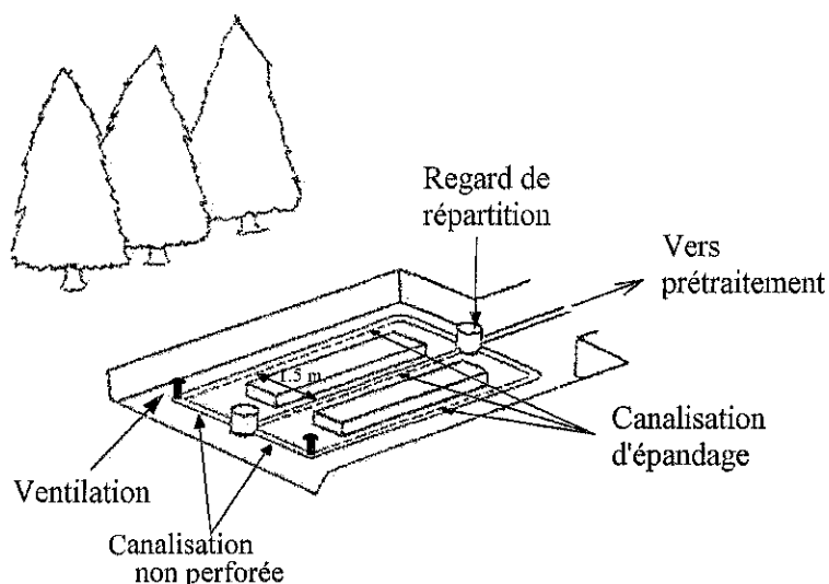
Schéma type du dispositif de traitement
